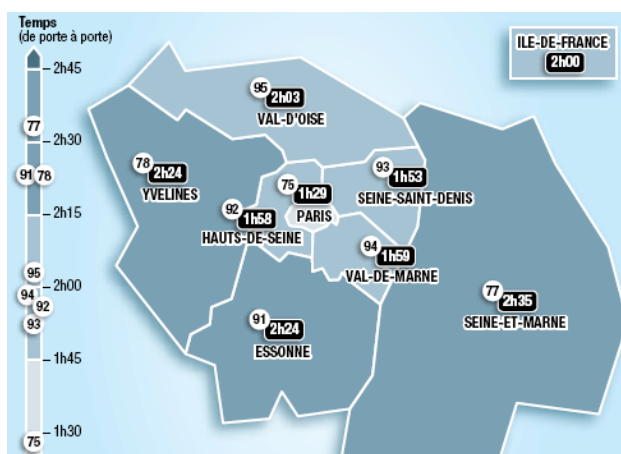
Temps de déplacement moyen en Ile-de-France -2011
